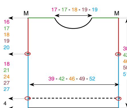
Patron du devant
