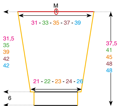
Patron des manches
