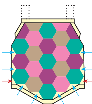
Schéma d'assemblage devant
