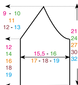
Patron demi-devant droit
