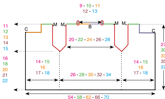
Patron du dos et des demi-devants
