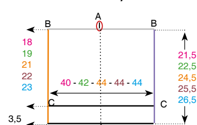
Patron de la capuche
