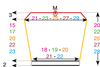
Patron de la capuche
