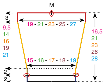
Patron des manches
