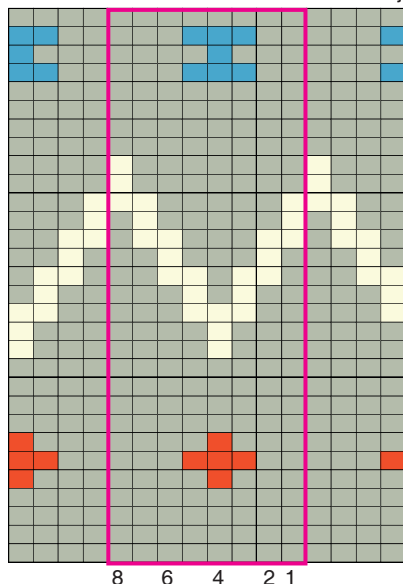
Diagramme jacquard
