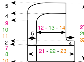
Patron cagoule assemblée (sauf bande finitions pour lien)
