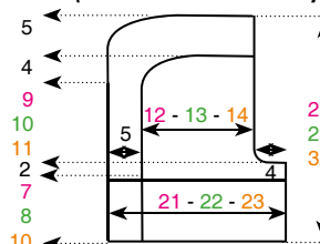
Patron cagoule assemblée (sauf bande finitions pour lien)
