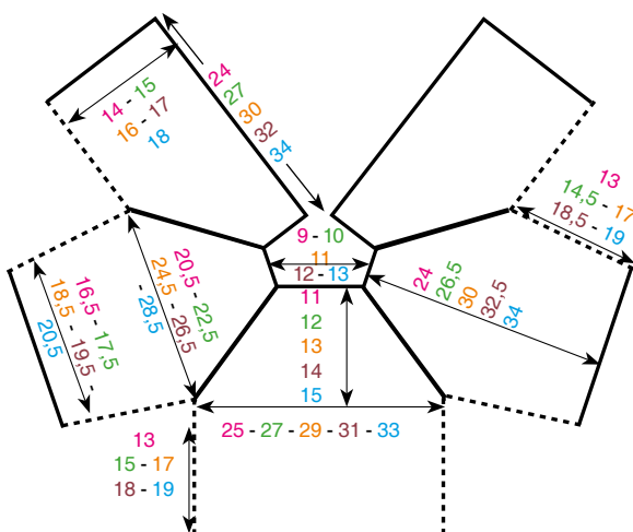
Patron corps et manches
