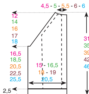
Patron manche droite
