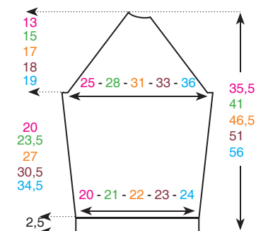
Patron manche droite
